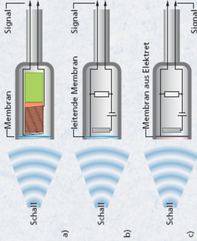
118.1 Funktionsweise von Mikrofonen a) dynamisches Mikrofon b) Kondensatormikrofon, c) Elektretmikrofon
